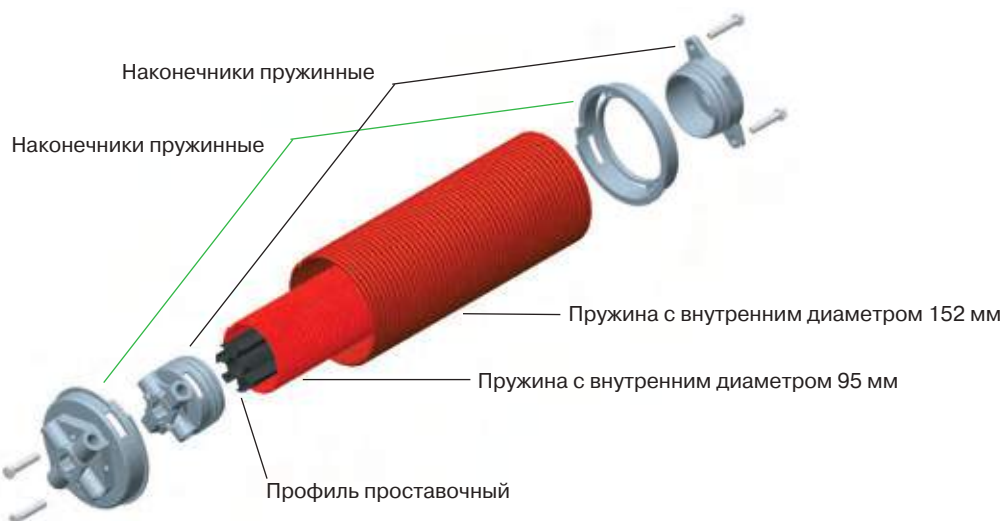
СХЕМАТИЧЕСКОЕ ИЗОБРАЖЕНИЕ ДУПЛЕКСНОЙ ПРУЖИНЫ
