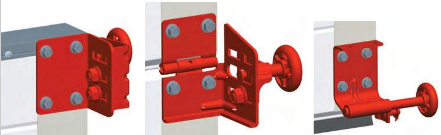
Кронштейн верхний
