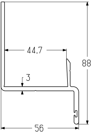
Обрамление калитки
