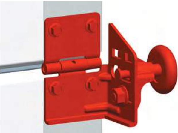
Кронштейн боковой
