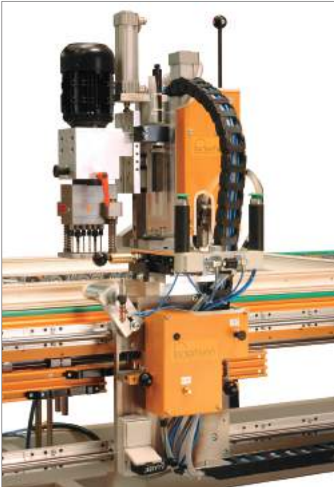
Две направляющие длиной 3200 мм для крепления сверлильного агрегата и шуруповёрта.
